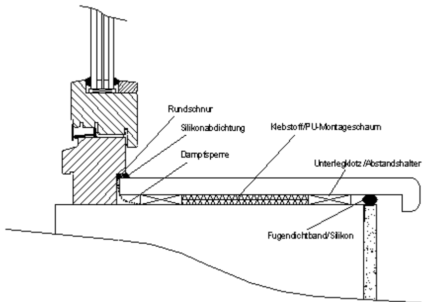
Abb. 8: Prinzipskizze einer eingebauten Fensterbank mit Dampfsperre
