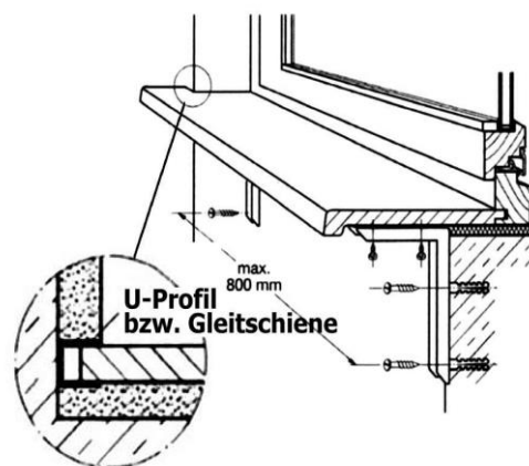
Abb. 7: Montierte Fensterbank mit am Fensterblendrahmen eingefräster Nut und seitlicher Befestigung in einem L- oder U- Profil
