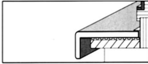
Abb. 13: Mit dem Untergrund vollflächig geklebte Fensterbank
