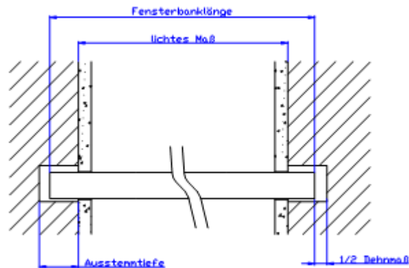
Abb. 11: Maßbezeichnungen für den Einbau einer eingeputzten Fensterbank
