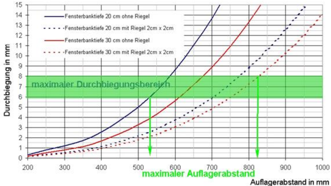
Diagramm 1: Durchbiegung bei mittiger Punktlast mit 1000 N
