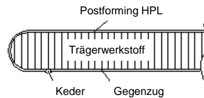
Abb. 2: Fensterbank mit Postformingprofil und Kederabdichtung
