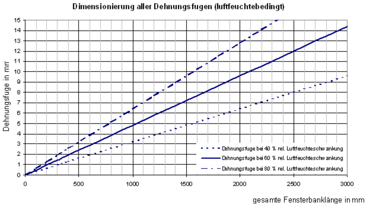
Diagramm 3: Dehnungsfugendimensionierung unter Berücksichtigung der durch Feuchtigkeit hervorgerufenen Längenausdehnung
