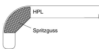
Abb. 6: Fensterbank aus HPL; Platte wird hinterfräst und mit Spritzgussmasse nach dem Verformen ausgegossen
