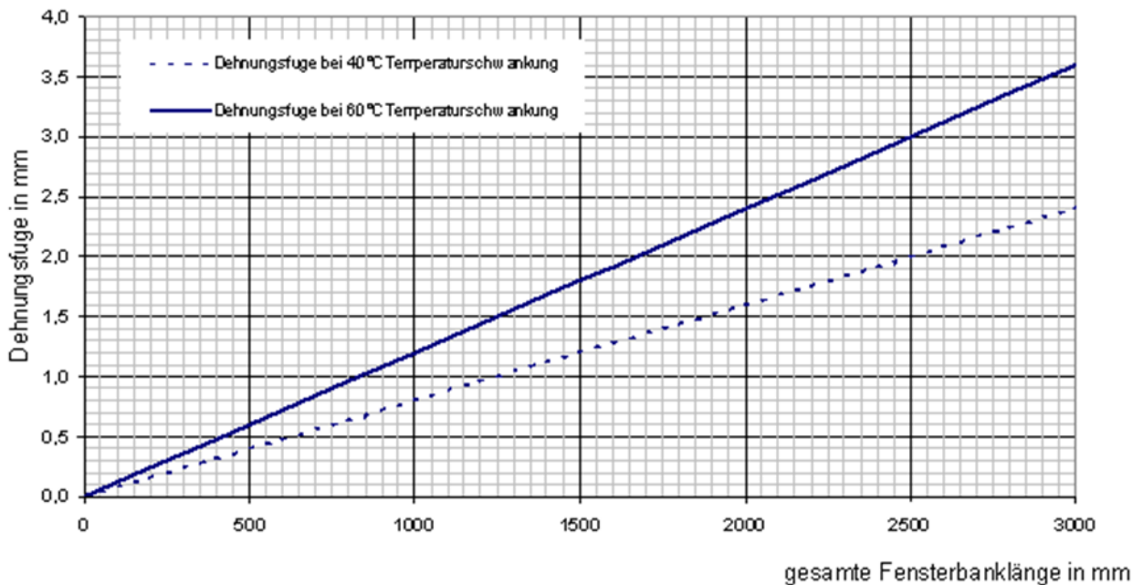
Diagramm 2: Ermittlung der Dehnungsfuge unter Berücksichtigung der thermischen Längenausdehnung
