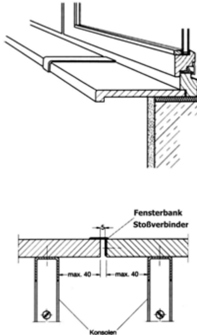
Abb. 10: Abdeckung der Plattenverbindung durch Profile
