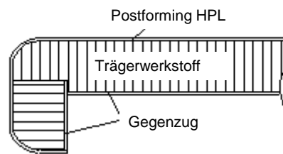
Abb. 1: Fensterbank mit Postformingprofilen und Abkantung
